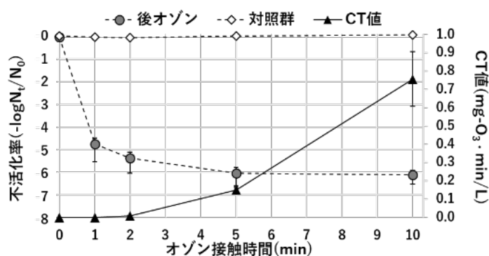
図-6 後オゾン処理の不活化特性
