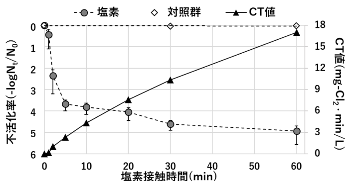
図-7 塩素処理の不活化特性
