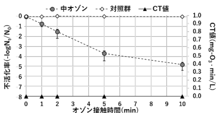
図-5 中オゾン処理の不活化特性
