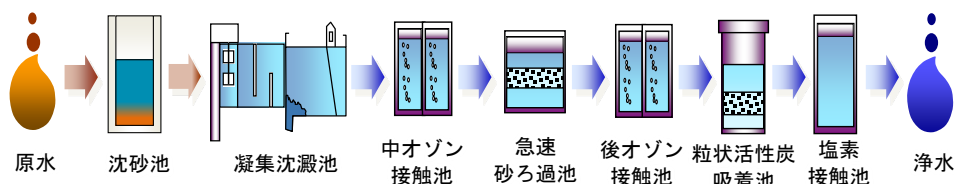
図-1 大阪市における浄水処理フロー
