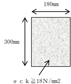
道路境界石数量表 (100m当り)
