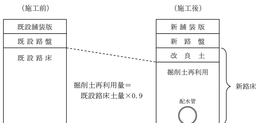
図2－1 掘削土再利用の考え方（変化率C＝0.90）
