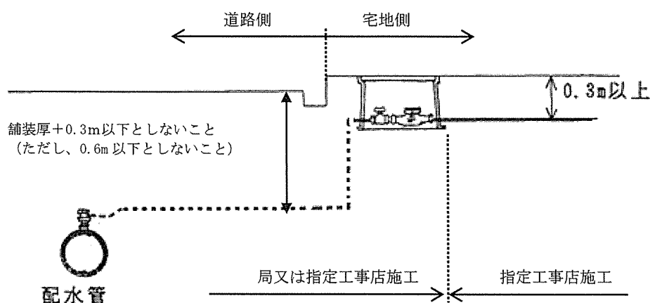
図2-36 宅地側からの分岐配管手順
