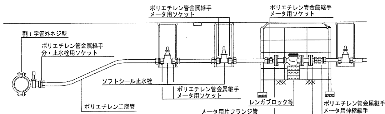
図 2-35 標準配管例
