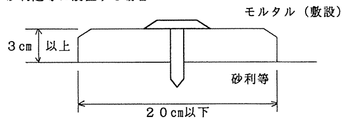
図 2-40 表示ピンの設置
