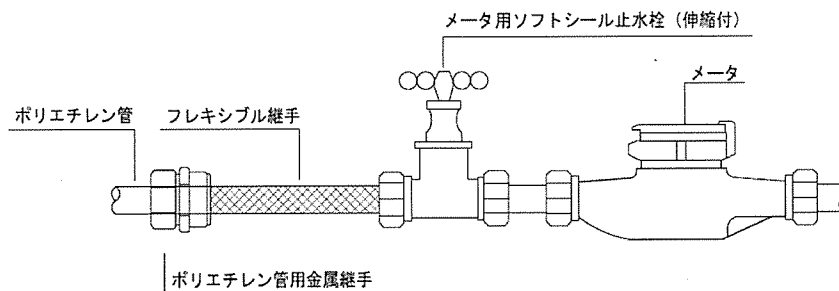
図 2-37 メータ流入側への設置例
