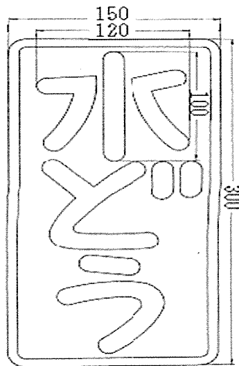
図2-34 水道マーク図（単位 mm）
