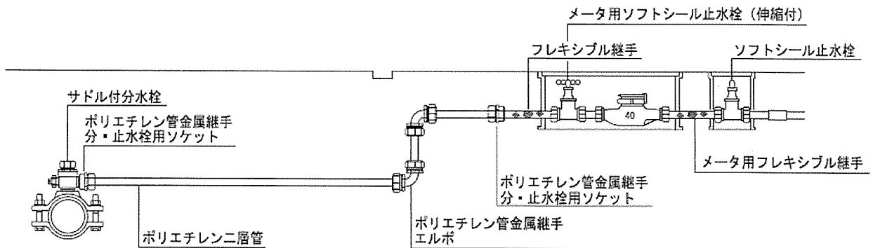
標準配管例（２）40mm（サドル付分水栓）
