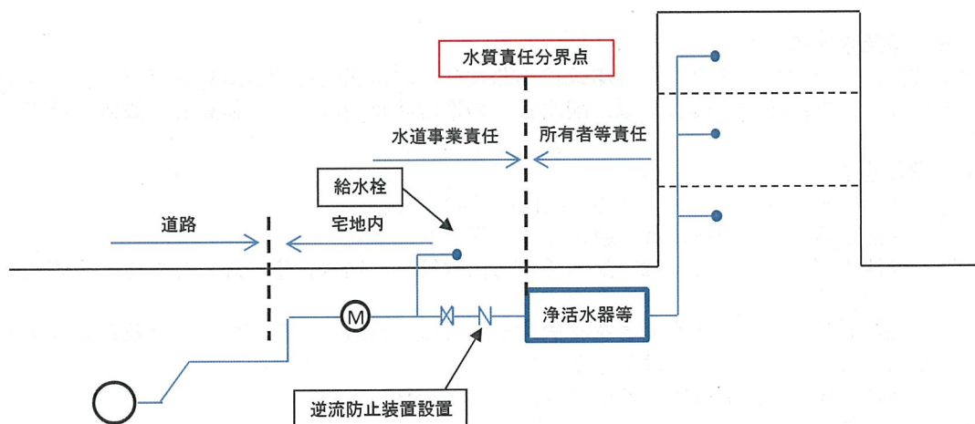
図 2-42 浄水器等の設置概略図
