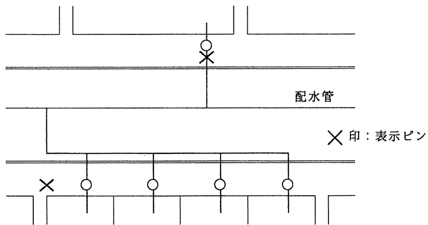
図 2-39 設置位置
