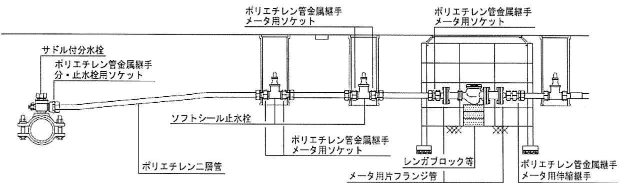
標準配管例（４）50mm（サドル付分水栓）
