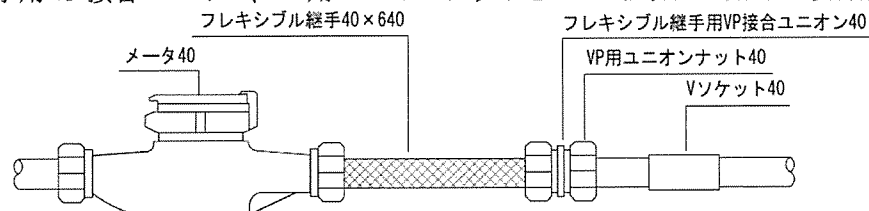
図 2-38 メータ内部側の止水栓を省略した場合の設置例
