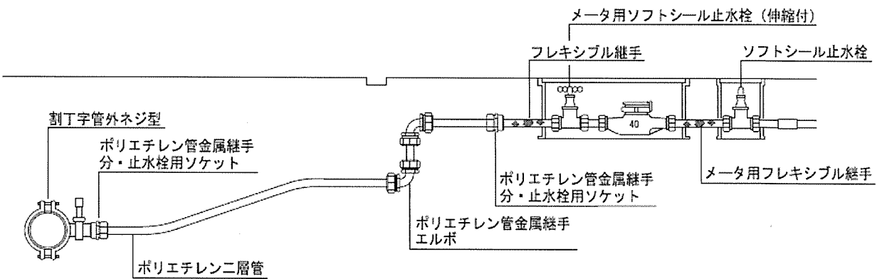
標準配管例（３）40mm（割Ｔ字管外ネジ型）
