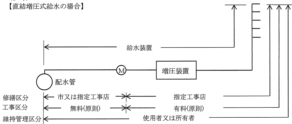
図 2-11 直結増圧式における維持管理区分
