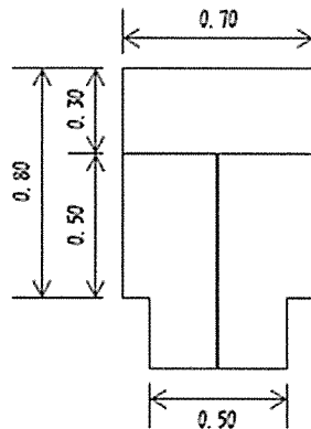
1 分水栓の場合
