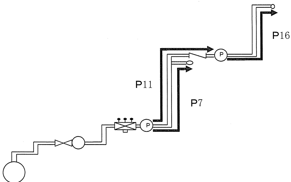
図 2-26 増圧装置設定圧力選択図
