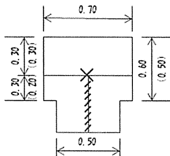
6 分水栓止めの場合 ( ) は、サドル付分水栓止めの場合
