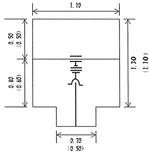
2 割T字管の場合 75 mm 以上 ( ) は、40・50 mm
