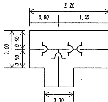
5 二受T字管の場合
