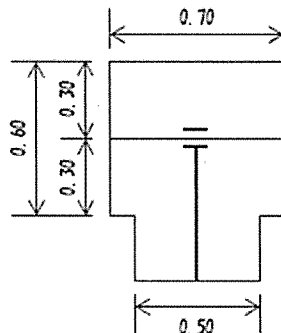
4 サドル付分水栓の場合 (25・40・50 mm )
