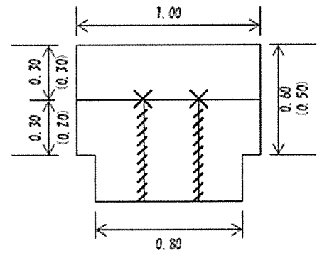
10 分水栓止め(2栓)の場合 ( ) は、サドル付分水栓止めの場合
