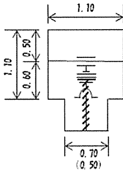
8 割T字管撤去・ 断水を伴う弁撤去の場合 75mm以上 ( ) は、40・50mm
