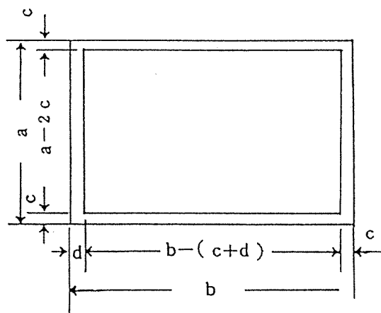
図2-27 図面の輪郭
