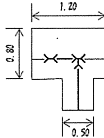
9 チーズ撤去の場合
