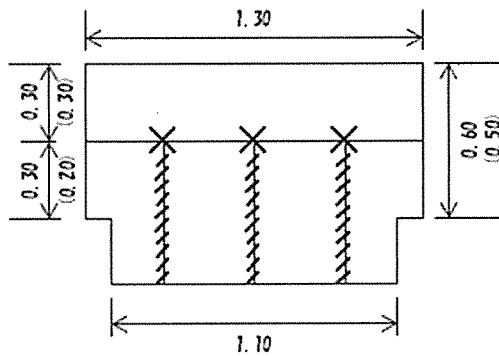
11 分水栓止め(3栓)の場合 ( ) は、サドル付分水栓止めの場合
