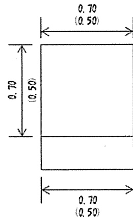
13 既設管接続の場合 75mm以上 ( ) は、50mm以下
