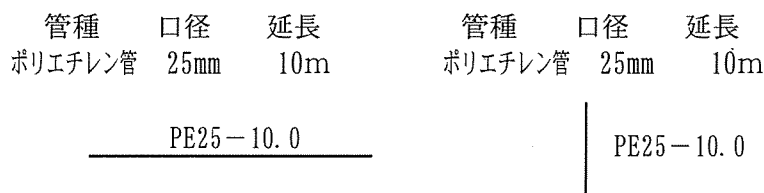
図2-28 給水管の表示(その1)
