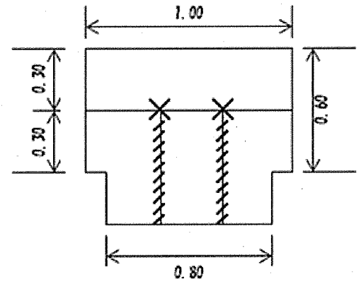
10 分水栓止め (2栓) の場合 または、サドル付分水栓止めの場合
