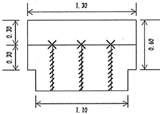
11 分水栓止め (3栓) の場合 または、サドル付分水栓止めの場合
