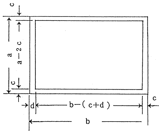
図2-27 図面の輪郭
