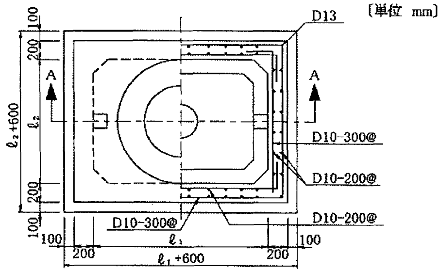
平面図
