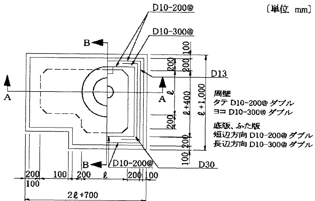
平面图
