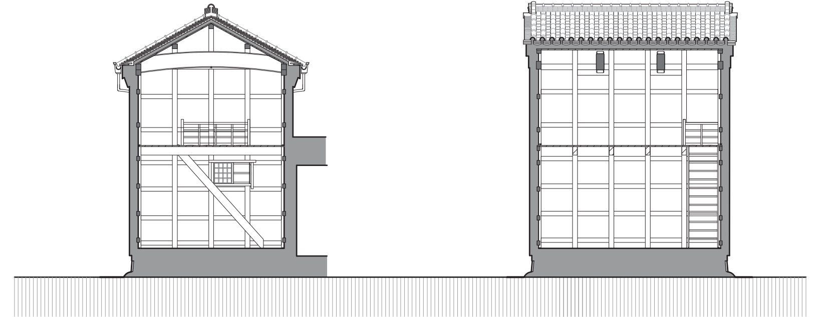
南北断面図
