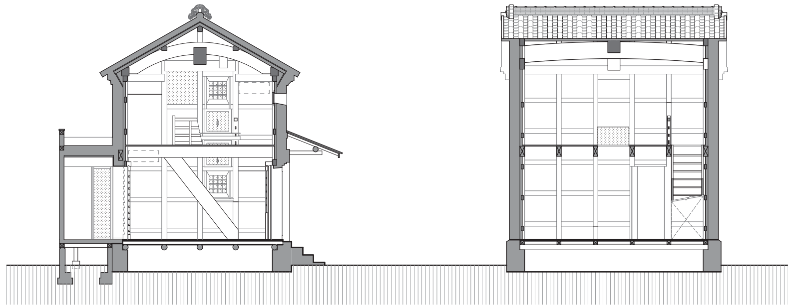
南北断面図
