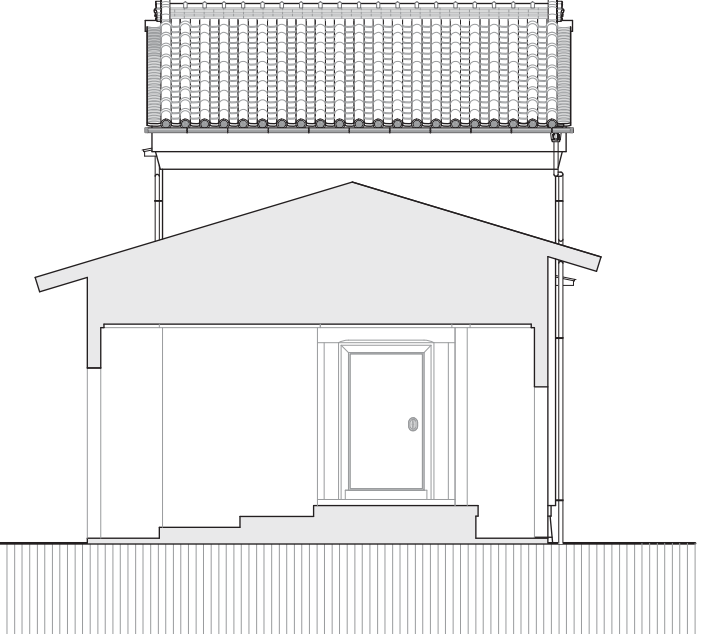
南立面図
