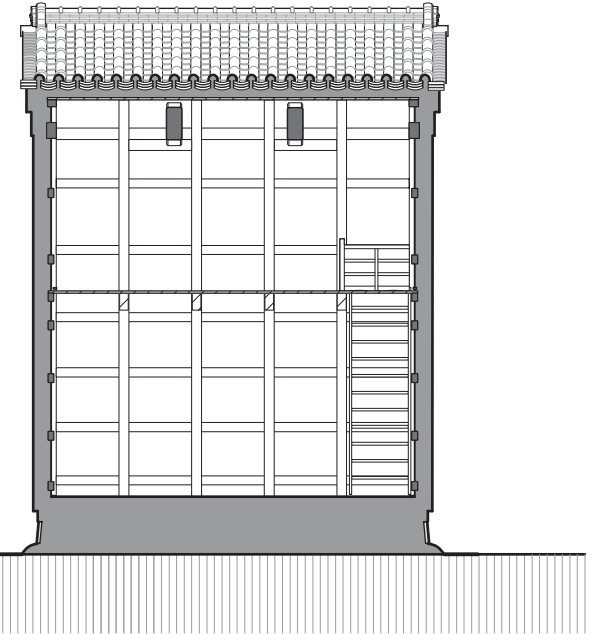
東西断面図
