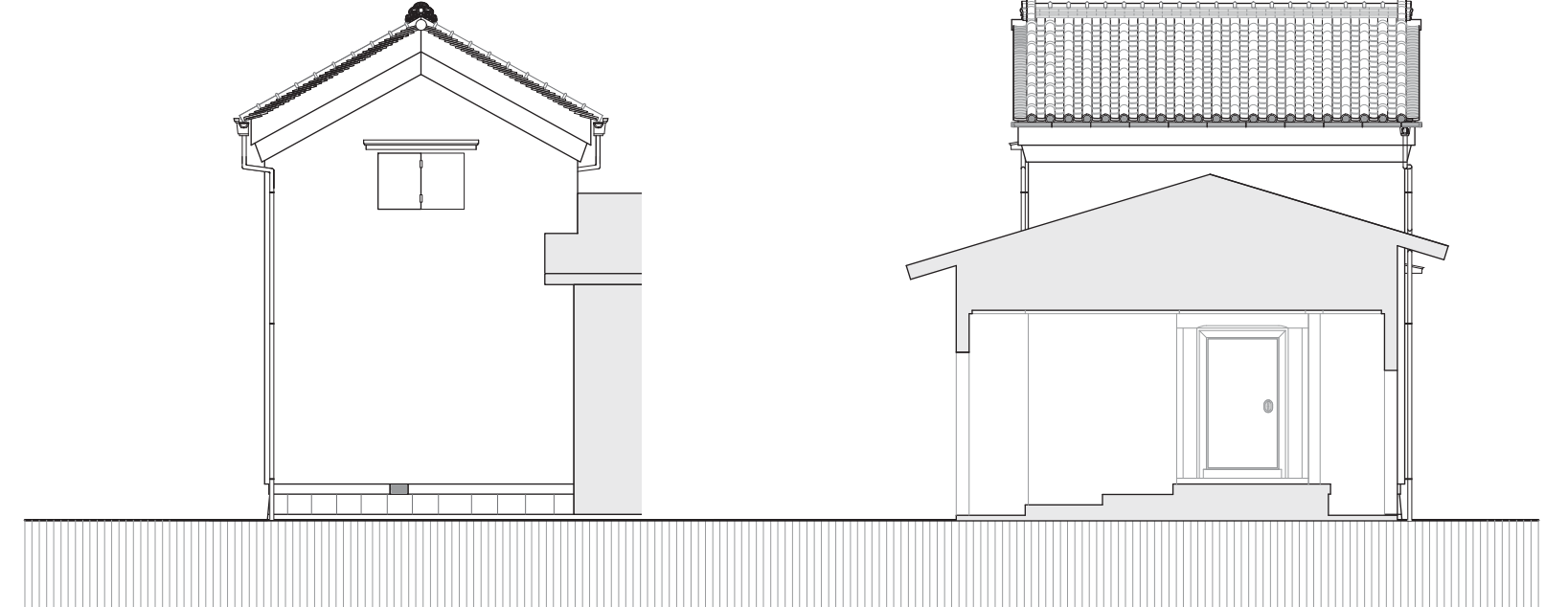
西立面図
