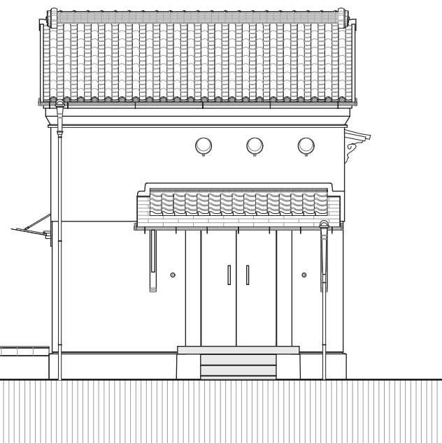
南立面図
