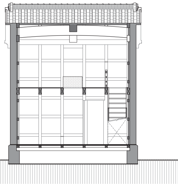
東西断面図
