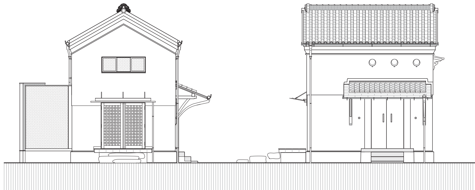
西立面図
