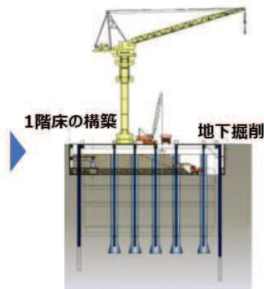
②基礎・躯体工事
