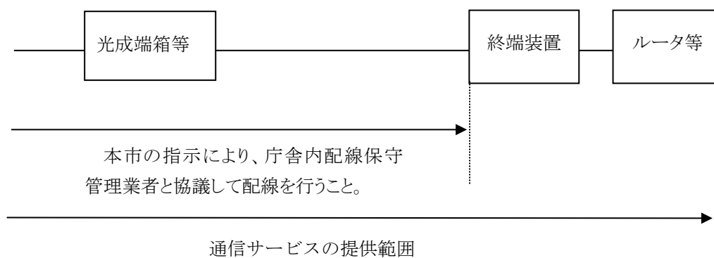
図 1-1 責任分界点
