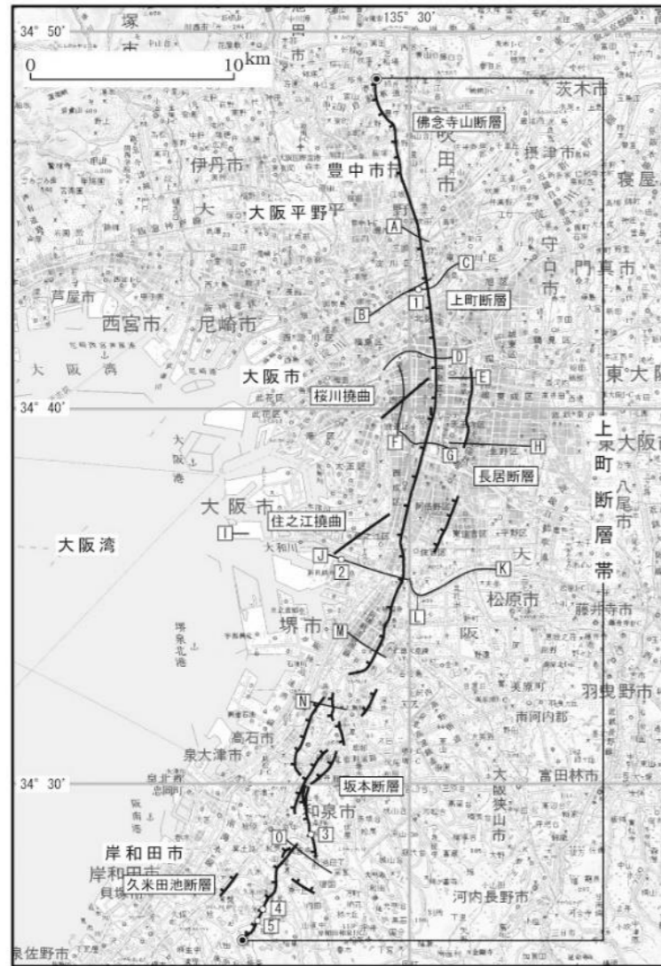
図 市域の活断層
