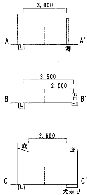
断面図 S = 1 / ○○○
