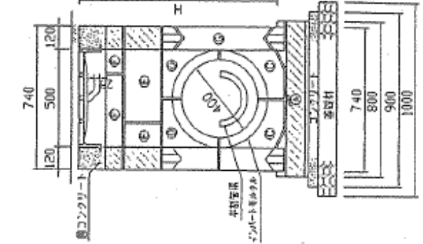
A-A' 断面図
