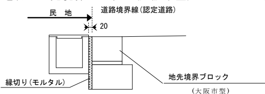
図 1-2 民地内歩道 標準仕様
