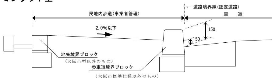
図 1-2 民地内歩道 標準仕様
