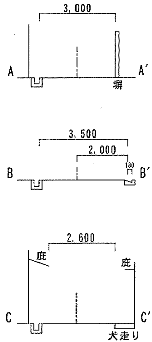
断面図 S = 1 / 〇〇〇
