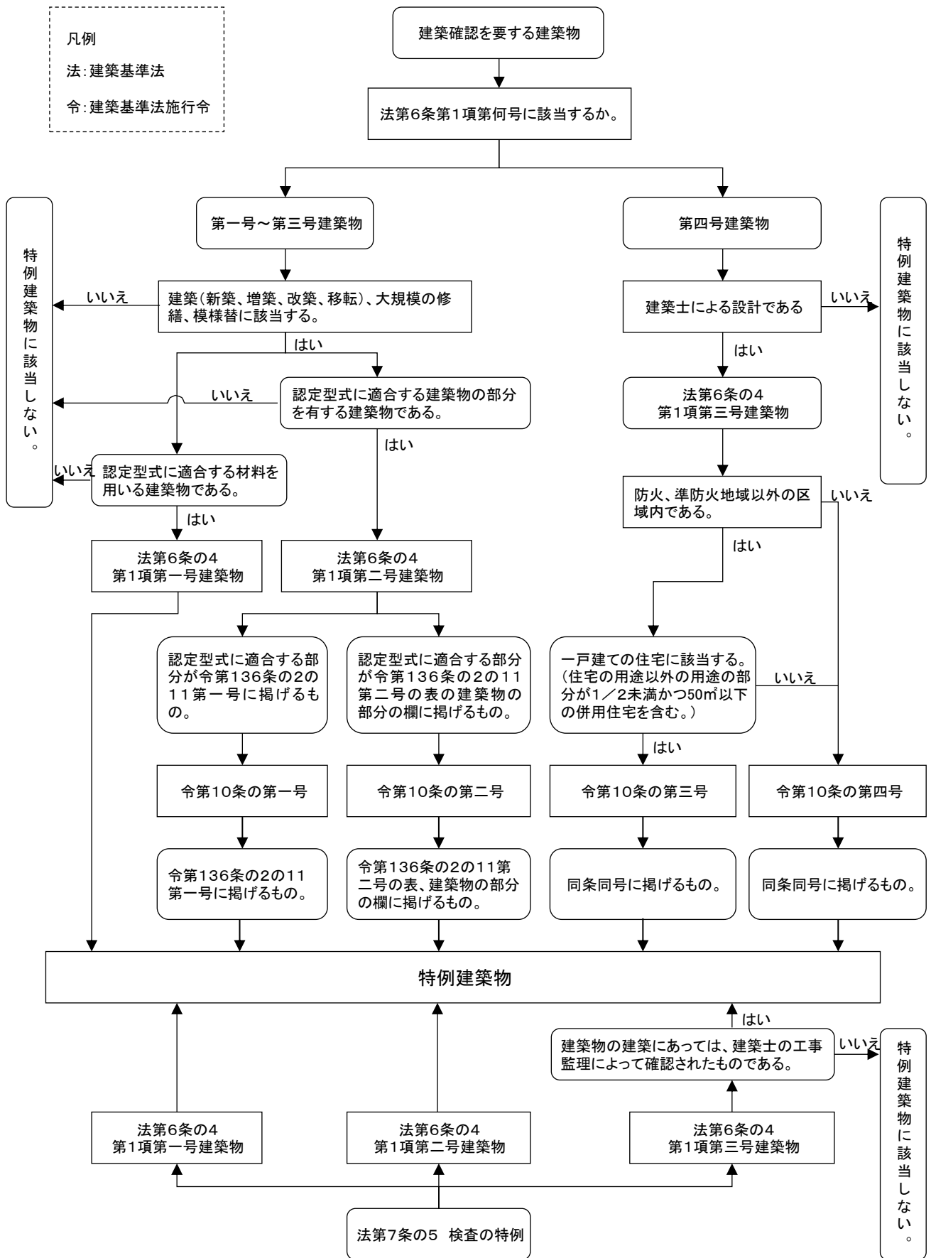
検査特例対象建築物判定フローチャート
