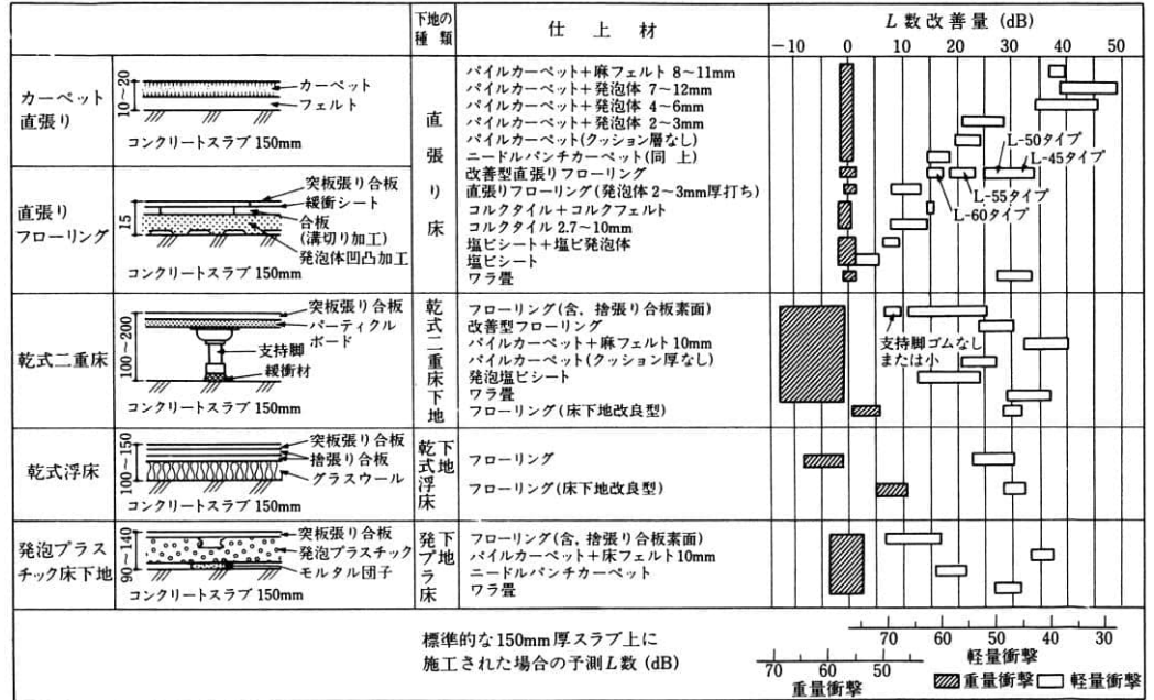
■参考2) 各種仕上げ材のL値改善量
