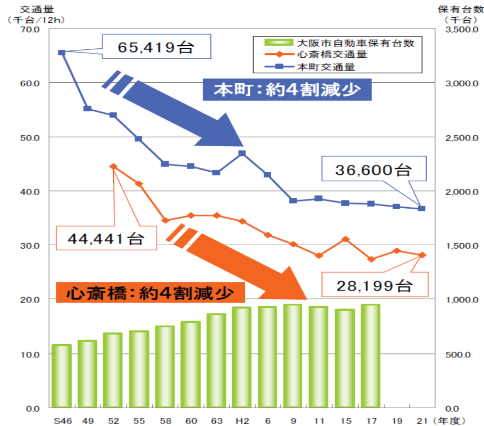
御堂筋における自動車交通の変遷
