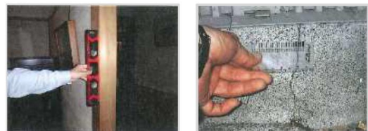
水平器による柱の傾きの計測
