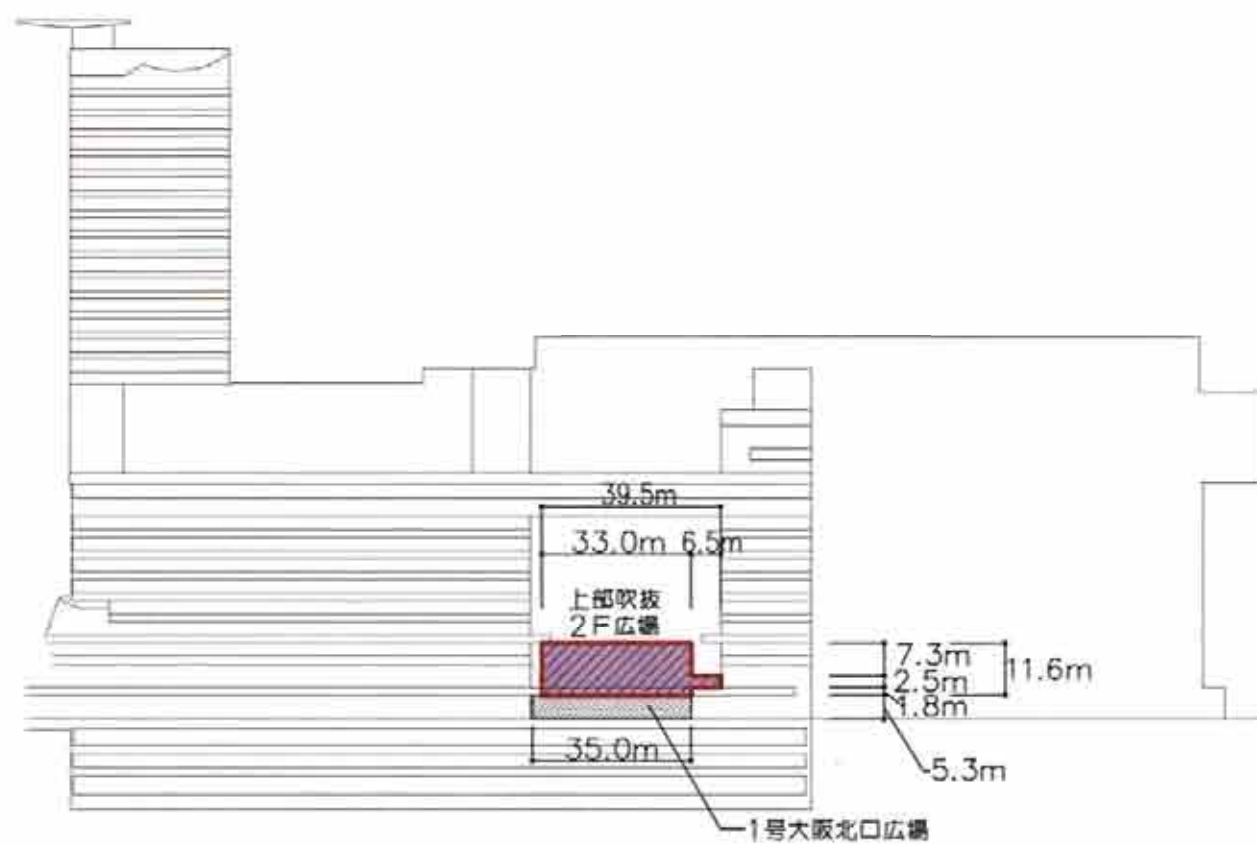
A-A断面図 1:1500
