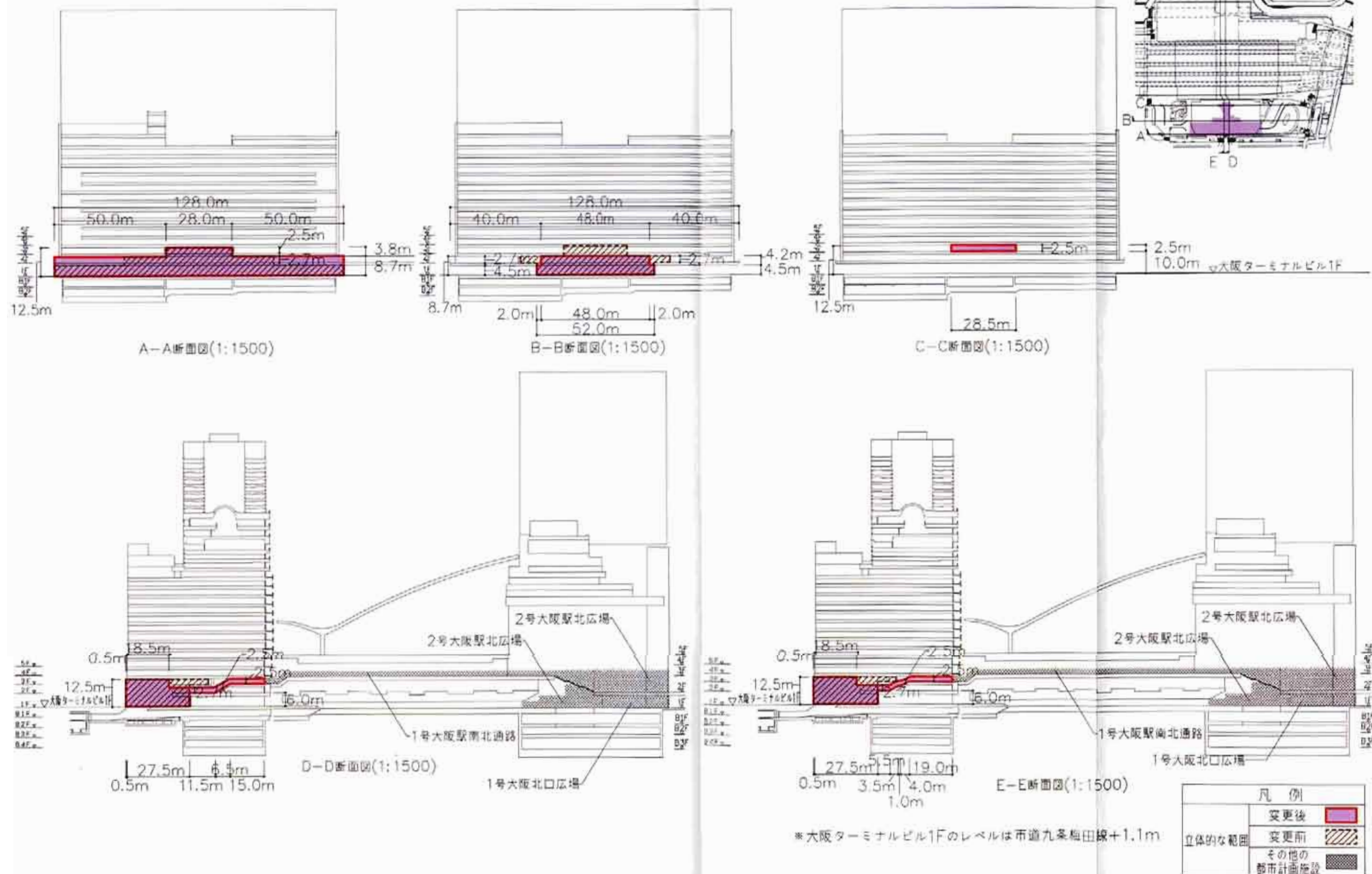
説明図3-2 交通広場（3号大阪駅南広場）断面図-1
