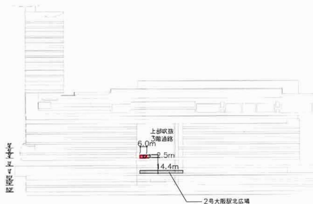
A-A断面図(1:1500)
