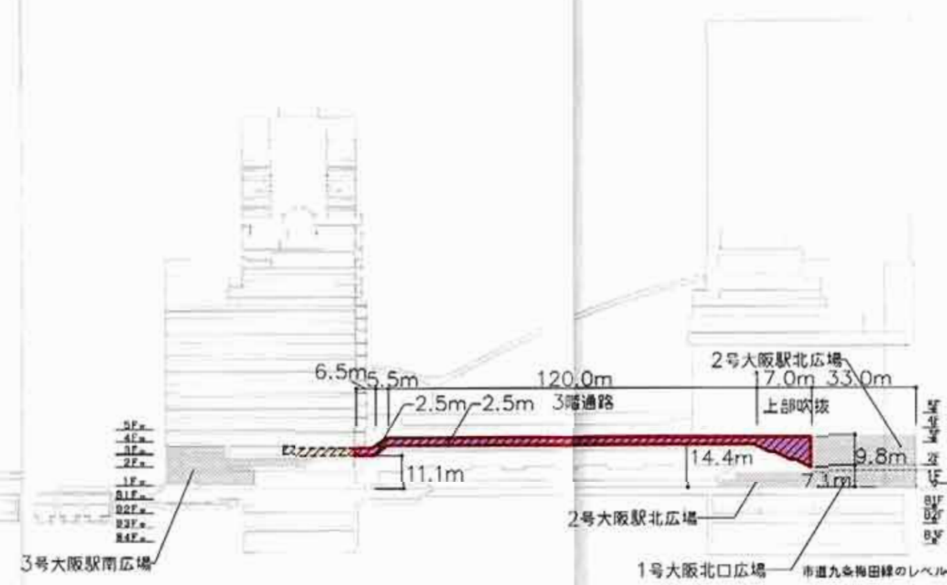
B-B断面図(1:1500)
