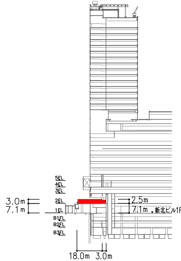
A-A断面図
