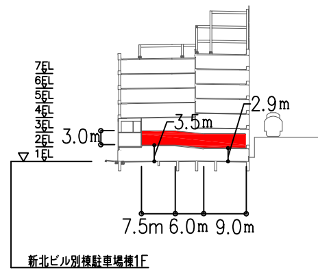
H-H断面図
