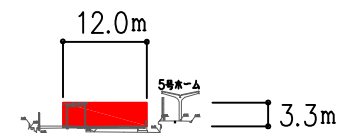
E-E断面図
