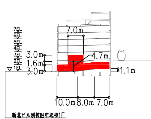
G-G断面図
