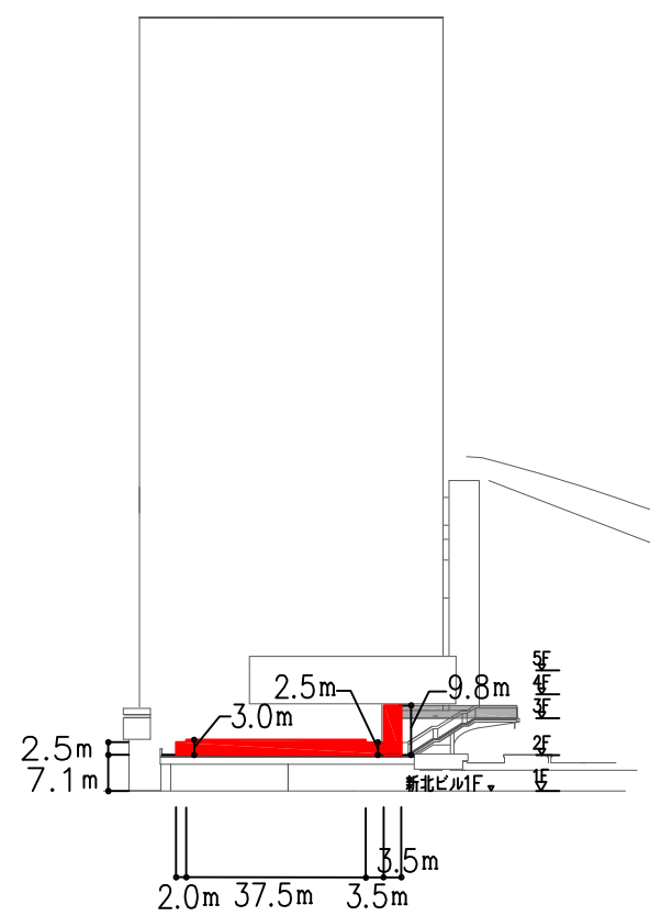
B-B断面図
