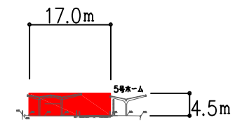
C-C断面図
