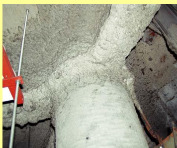
鉄骨耐火被覆材
