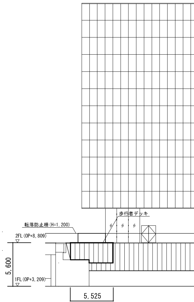
西立面図 1/300
