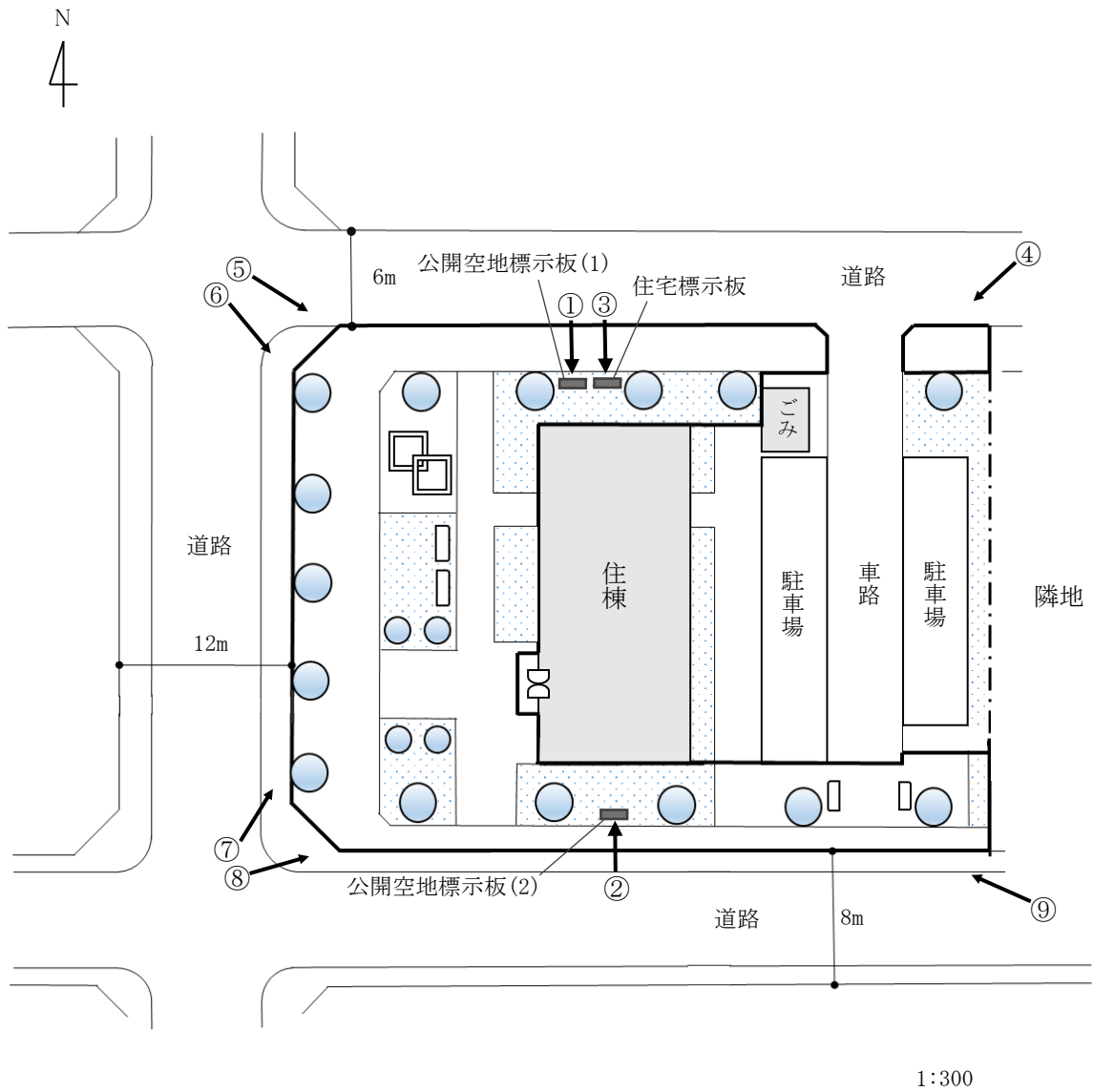
配置図兼公開空地平面図参考例
