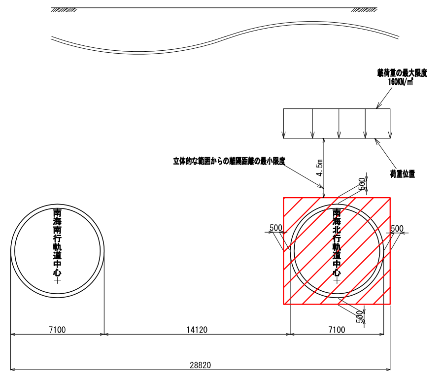
南海新難波～新今宮 単線シールド区間 4k850m
