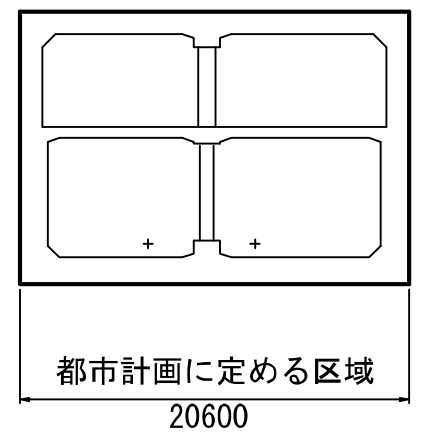
夢洲北線路部 断面⑤
