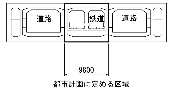
夢洲南線路部 断面③
