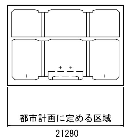
夢洲北線路部 断面⑤
