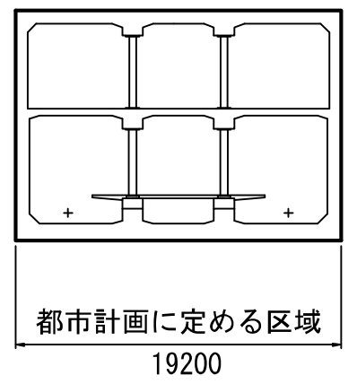
夢洲～車庫線部（線路縦断部） 断面⑥
