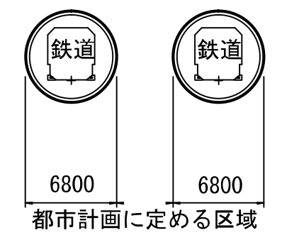
夢洲駅部 断面④
