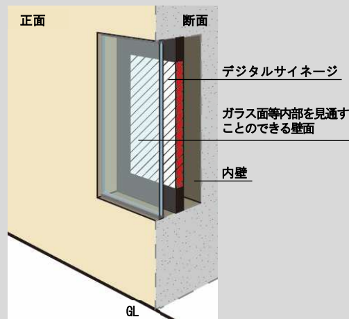
ガラス面等より内側※に設置された広告物の例 (正面図+断面図)
