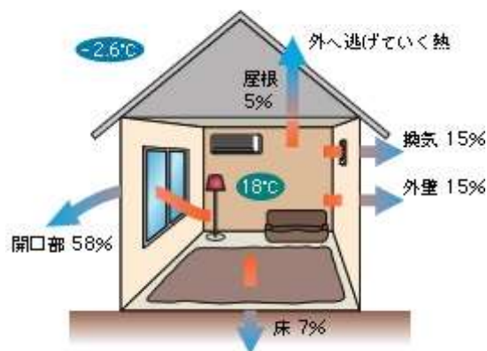
■冬の暖房時の熱が開口部から流失する割合 58%
