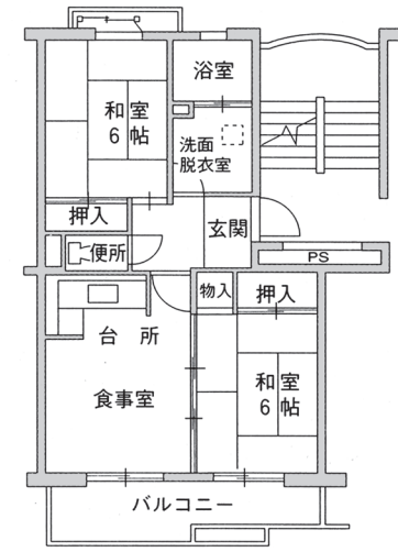
2DKタイプ (住居専用面積 53m 2 ) (バルコニー面積 9m 2 )
