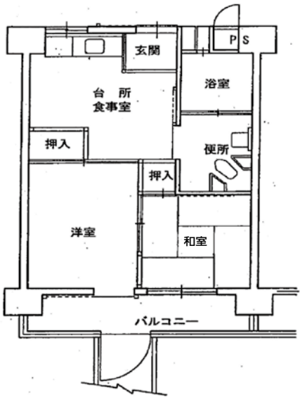
車いす常用者向特別設計住宅の間取図(例)
