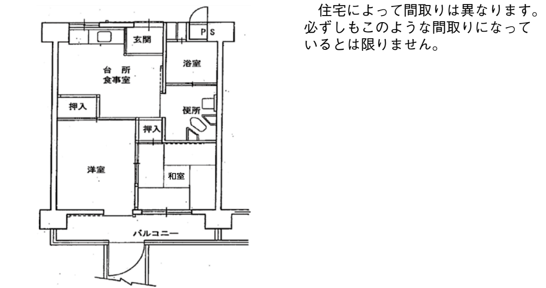
車いす常用者向特別設計住宅の間取図(例)
