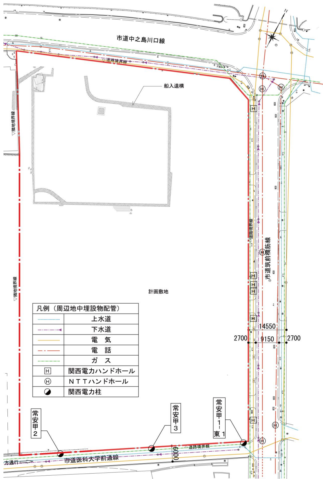
道路の埋設管状況
