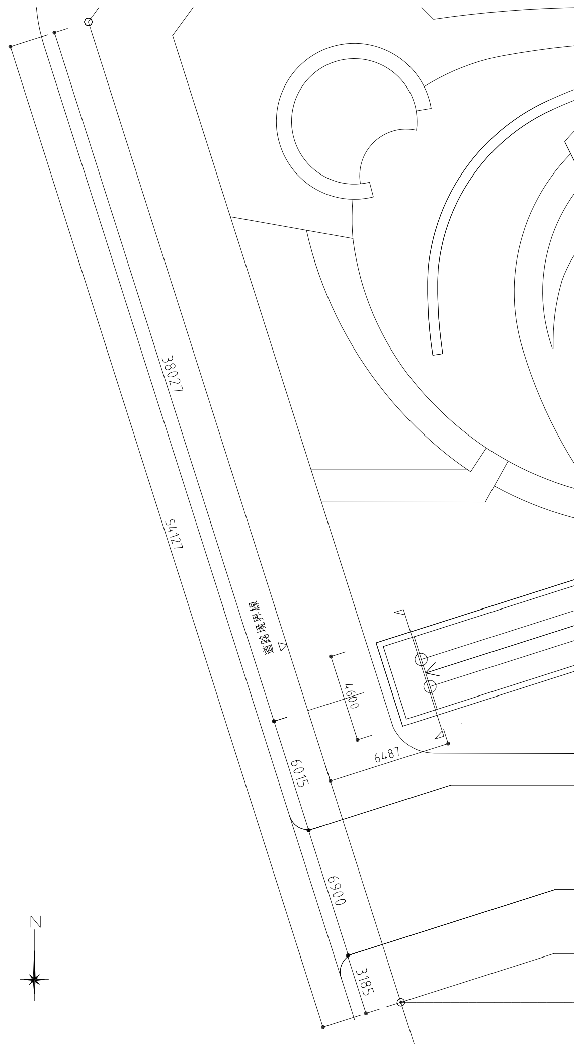
北東デッキ平面図 1/200
