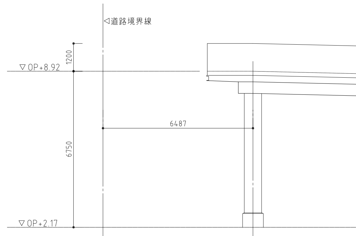
北東デッキ立面図 1/100
