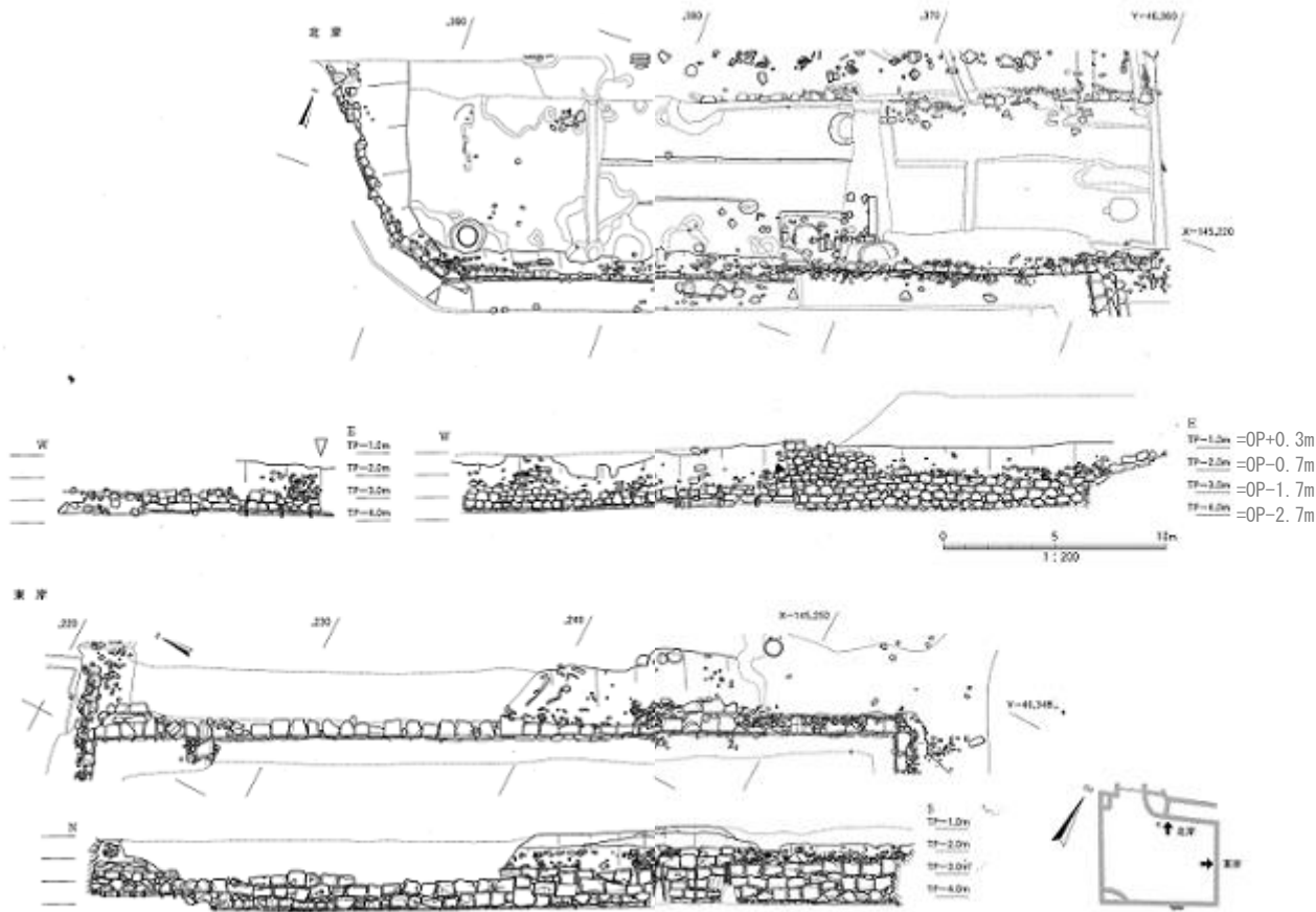
図27 「船入JSF2001平面・立面図(1)」
