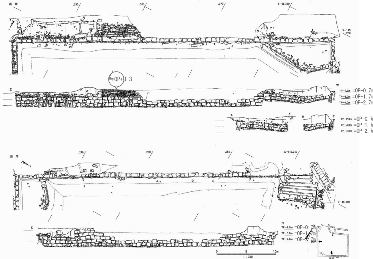
図28 「船入JSF2001平面・立面図(2)」
