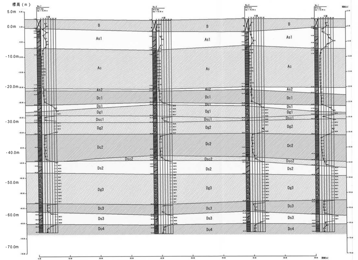
地層推定断面図(No. 7~No. 6~No. 3~No. 1)
