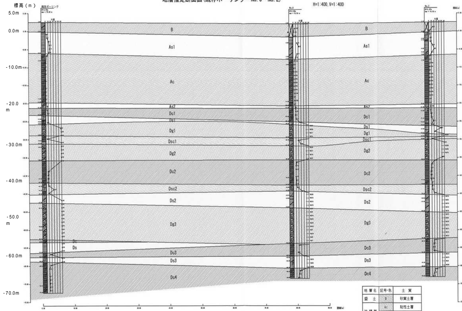
地層推定断面図(既存ボーリング~No. 6~No. 2)
