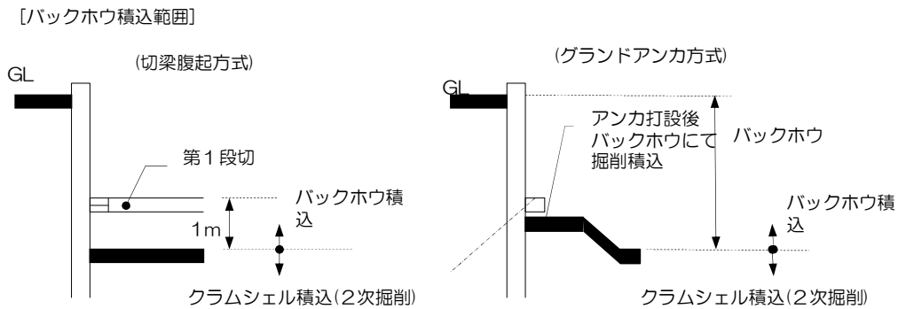
図1-3 根切りの分類とバックホウ積込範囲
