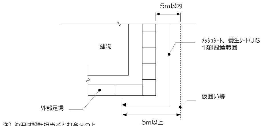
図1-2 スッポット、養生シート(JIS 1類)等設置範囲(参考)
