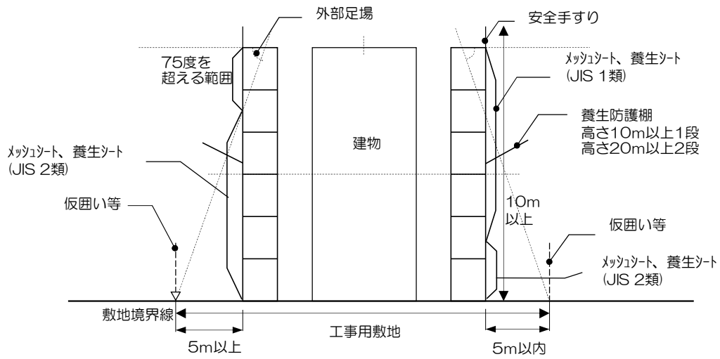
図1-1 災害防止設置要領(参考)
