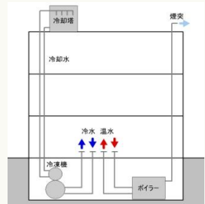
冷凍機＋ボイラー方式
