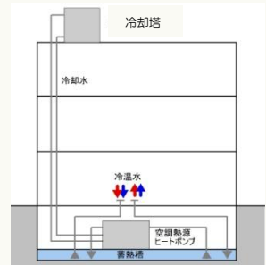
ヒートポンプ＋蓄熱槽方式
