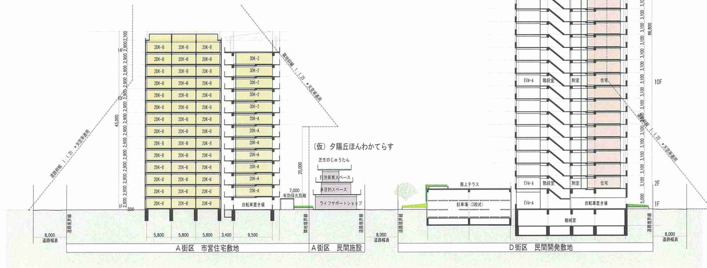
A-D街区 南北断面図
